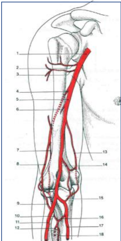
Figure 01 : artère brachiale
